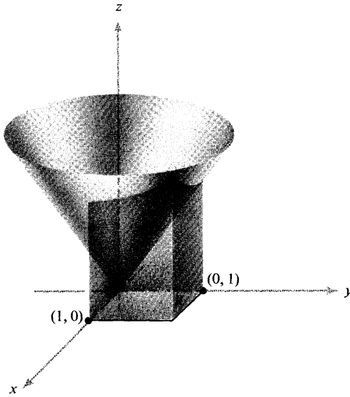
Figura 6.3.9 Volumen de la región bajo z = \sqrt{x^2 + y^2} y sobre R = [0, 1] \times [0, 1] .
